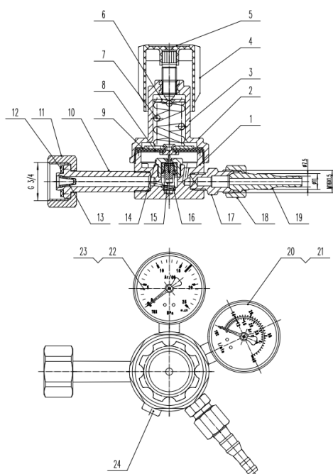
Рис. 1. Регулятор расхода газа баллонный одноступенчатый У30/AP40KP:
