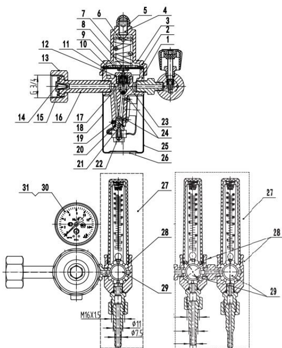
Рис. 5. Регулятор расхода газа баллонный одноступенчатый У 30/АР 40 КРП Р, У 30/АР 40 КРП Р2:
