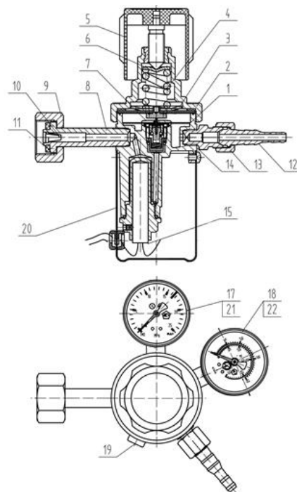
Рис. 4. Регулятор расхода газа баллонный одноступенчатый У 30 KP:
