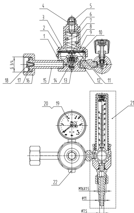
Рис. 2. Регулятор расхода газа баллонный одноступенчатый с У30/AP40KP-P:
