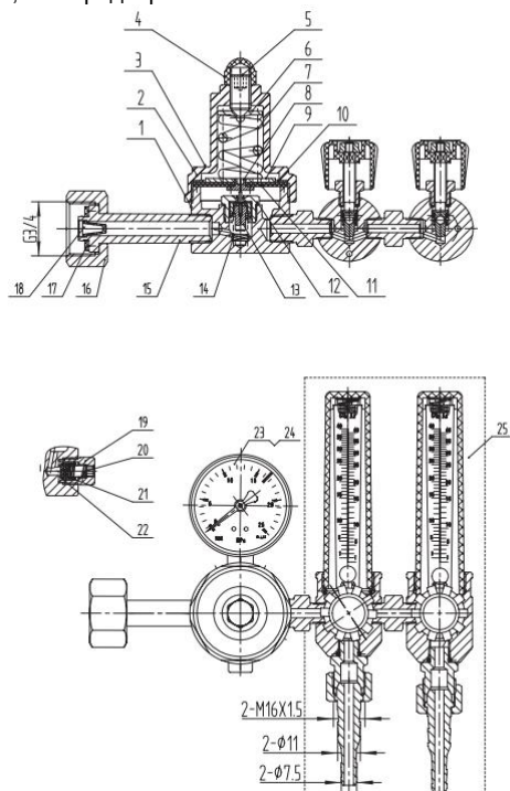
Рис. 3. Регулятор расхода газа баллонный одноступенчатый У 30 / AP40 KP P2:
